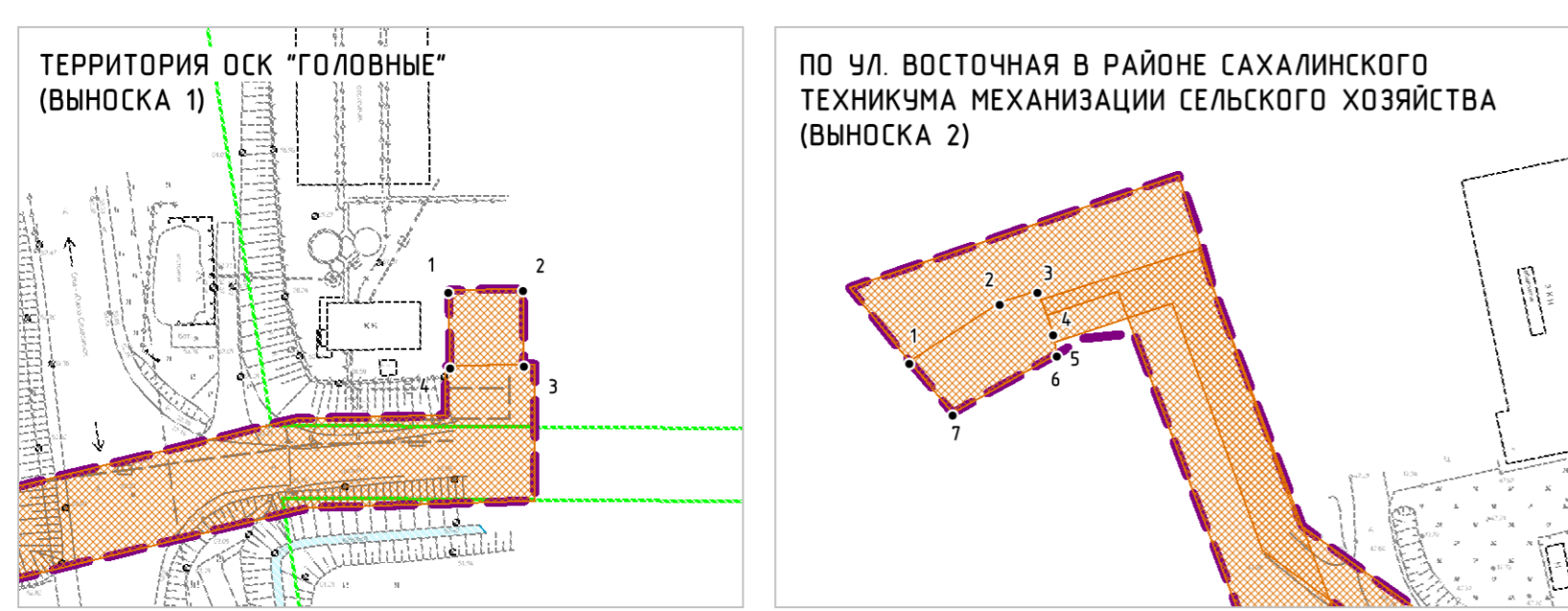
ЧЕРТЕЖ ГРАНИЦ ЗОН ПЛАНИРУЕМОГО РАЗМЕЩЕНИЯ ЛИНЕЙНЫХ ОБЪЕКТОВ, ПРОЕКТИРУЕМЫХ В СОСТАВЕ ЛИНЕЙНЫХ ОБЪЕКТОВ (КАНАЛИЗАЦИОННЫЕ НАСОСНЫЕ СТАНЦИИ) М 1:1 000
