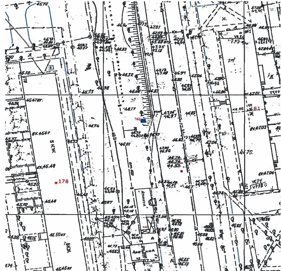
Топосъемка М 1:500
