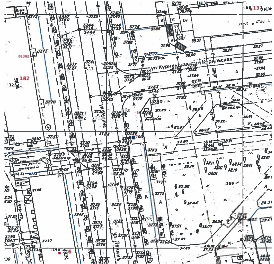
Топосъемка М 1:500
