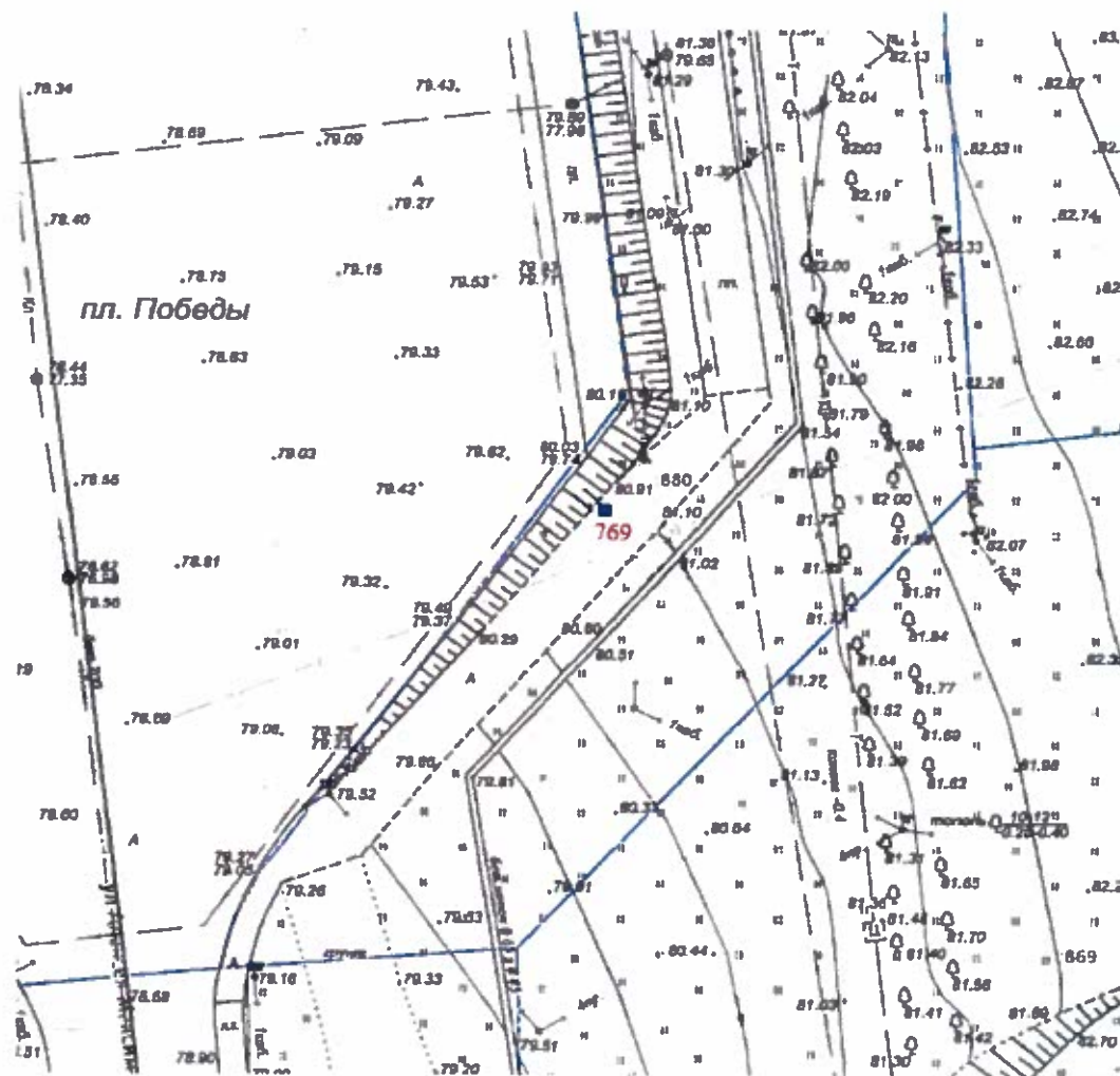
Топосъемка М 1:500
