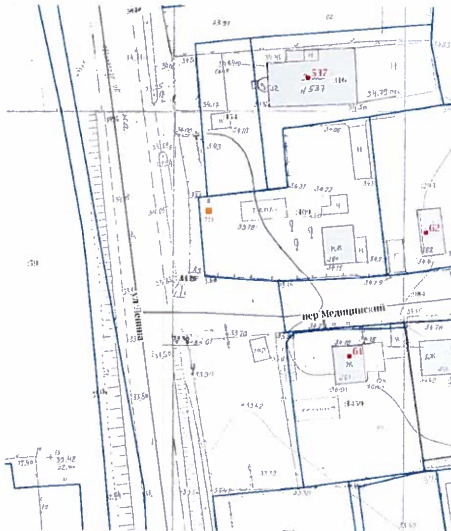
Топоъемка М 1:500
