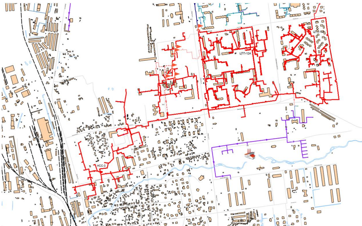
Рисунок 5.1 – Зона действия котельной «Южная» актуализированный вариант
