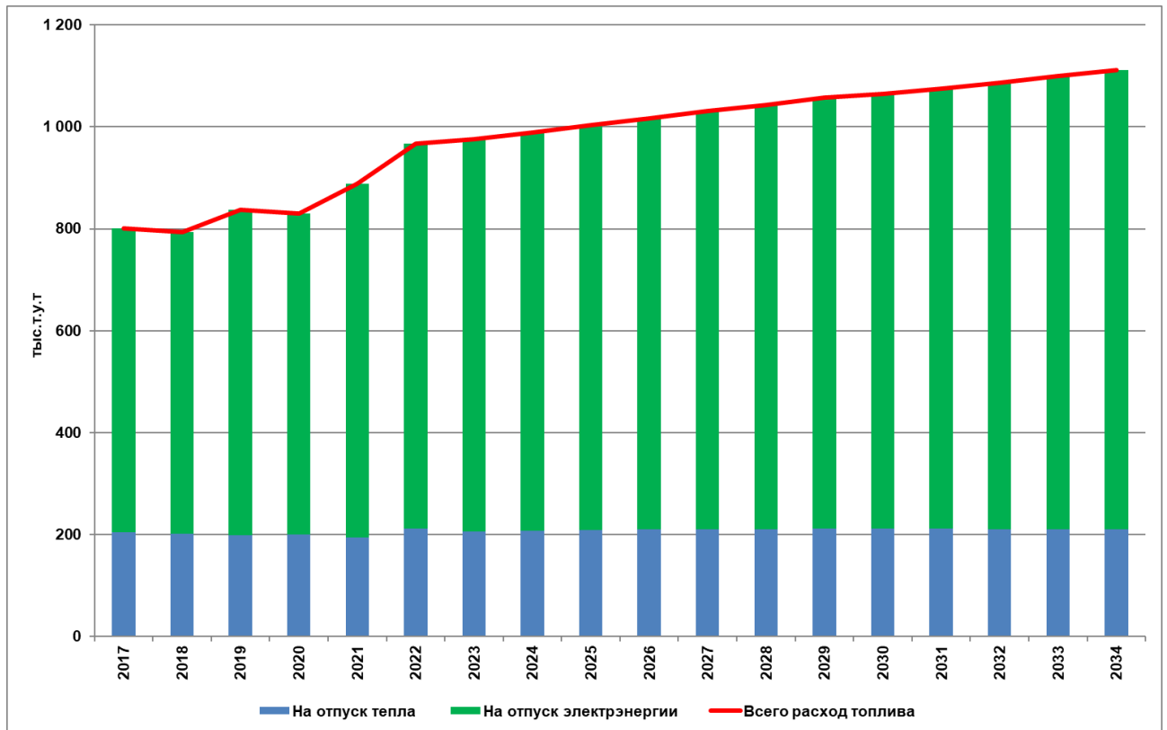
Рисунок 9.1 – Суммарное потребление топлива на выработку тепловой и электрической энергии на Ю-СТЭЦ-1 в 2017-2034 годах
