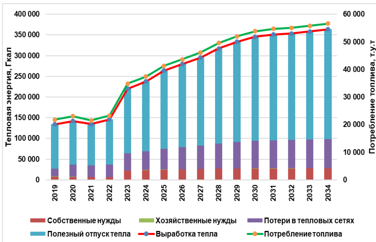
Рисунок 9.2 – Структура выработки тепловой энергии котельными АО «СКК» в 2019-2034 годах
