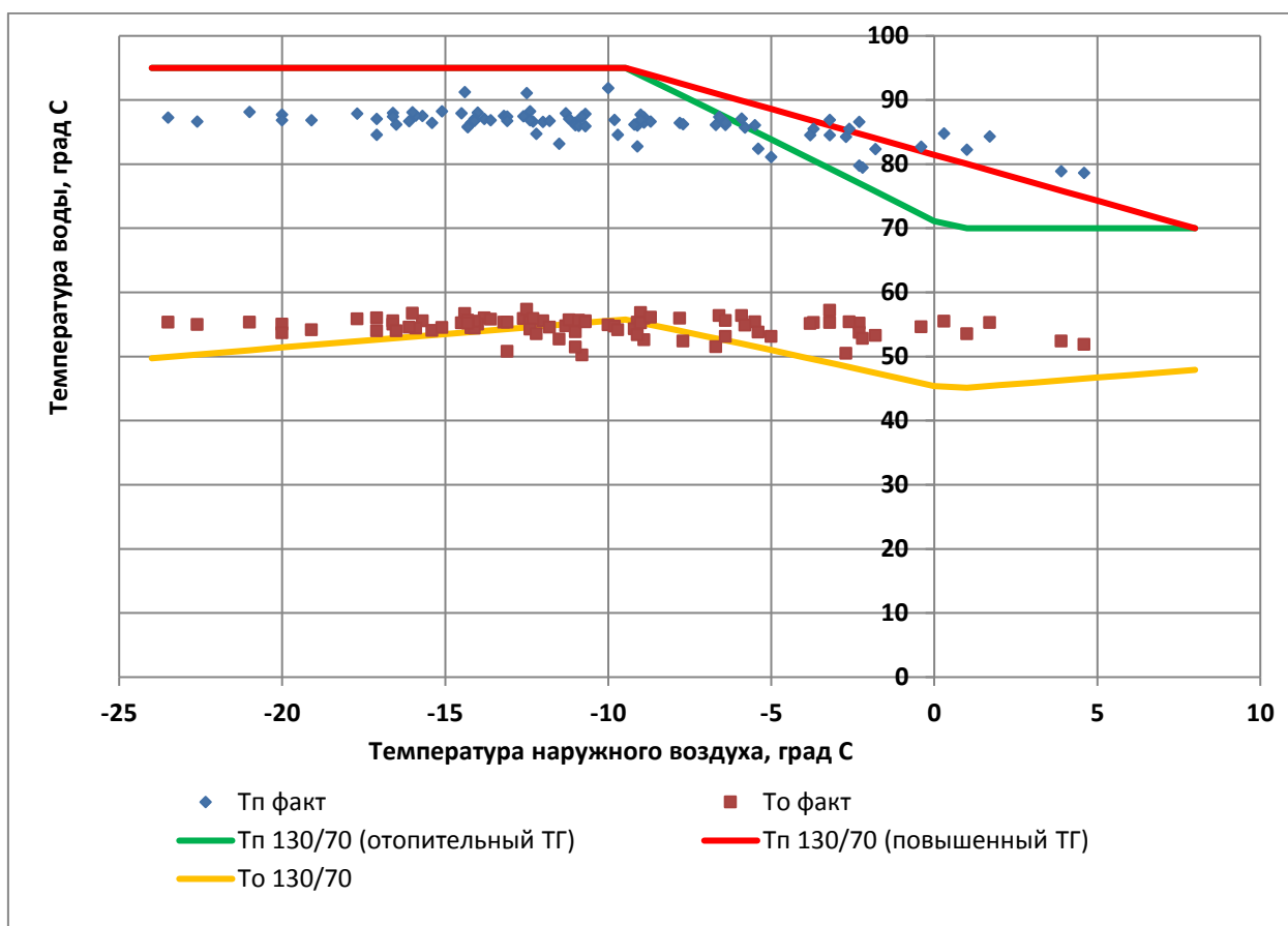
Рисунок 6.3 - Фактические температуры сетевой воды и температурные графики для теплового вывода
